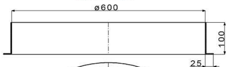
MAX RING
